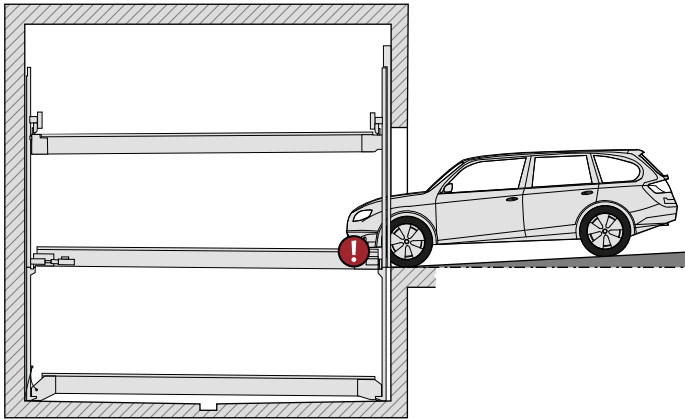
max. 3% Gefälle
