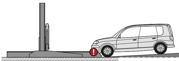
max. 4% Gefälle
